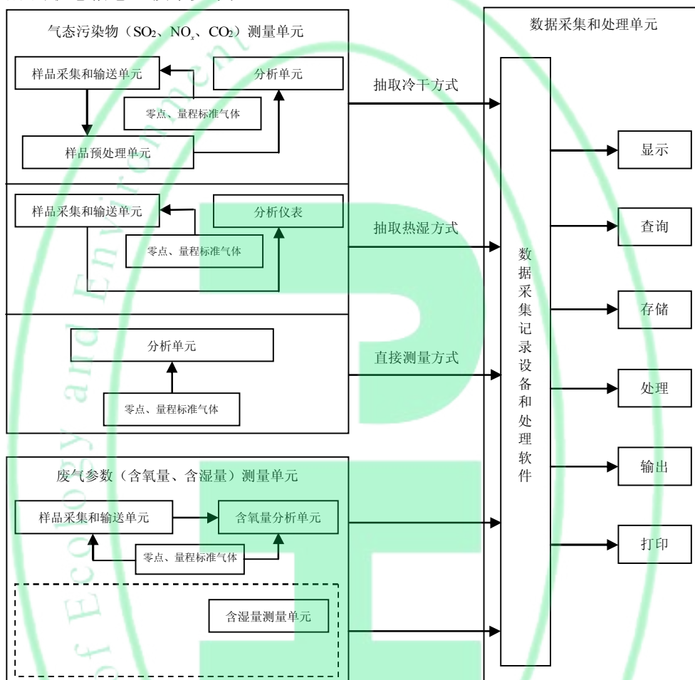
图 1 二氧化硫、氮氧化物和二氧化碳便携式红外吸收仪组成示意图
